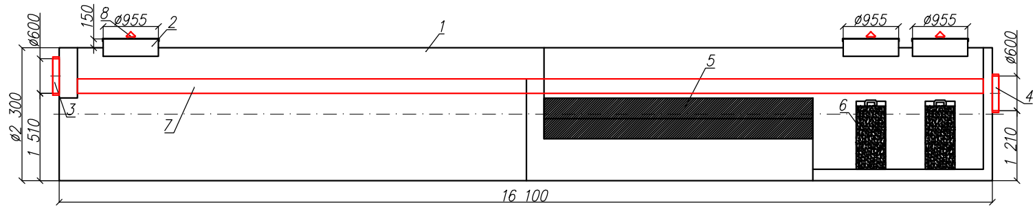
Разрез 1-1
